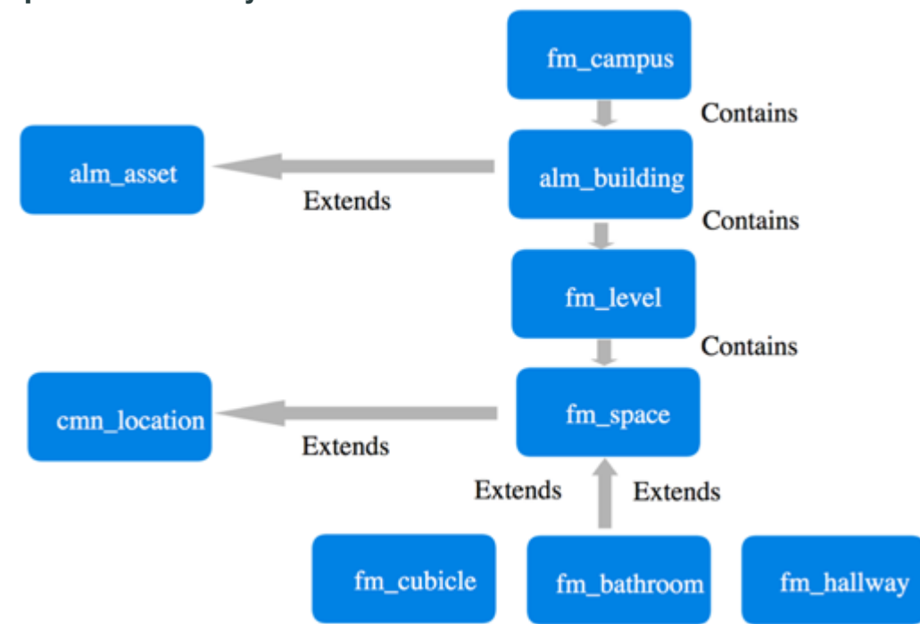
Space table hierarchy
