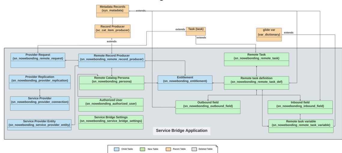
Modèle de données client de Service Bridge
