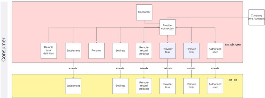
Modèle de données de Service Bridge for Consumers
